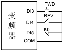
图 7-14-B 三线式运行模式 2
