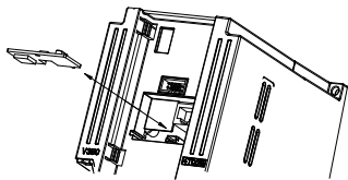
图 3-7-B II 类功能板的安装拆卸示意图
