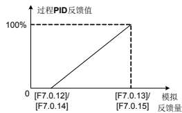
图 7-53 过程 PID 反馈值对应关系示意图
