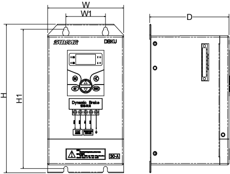
图 12-17 安装尺寸
