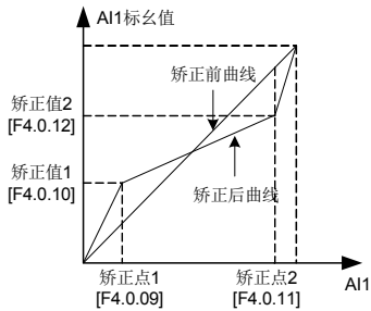
图 7-38 模拟输入 AI1 曲线
