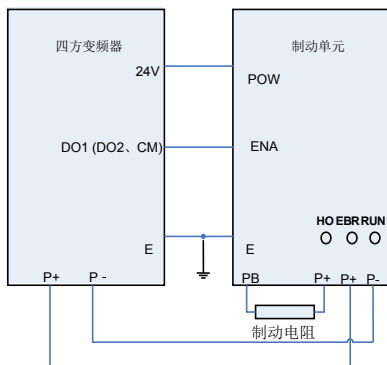
图 13-18 接线示意
