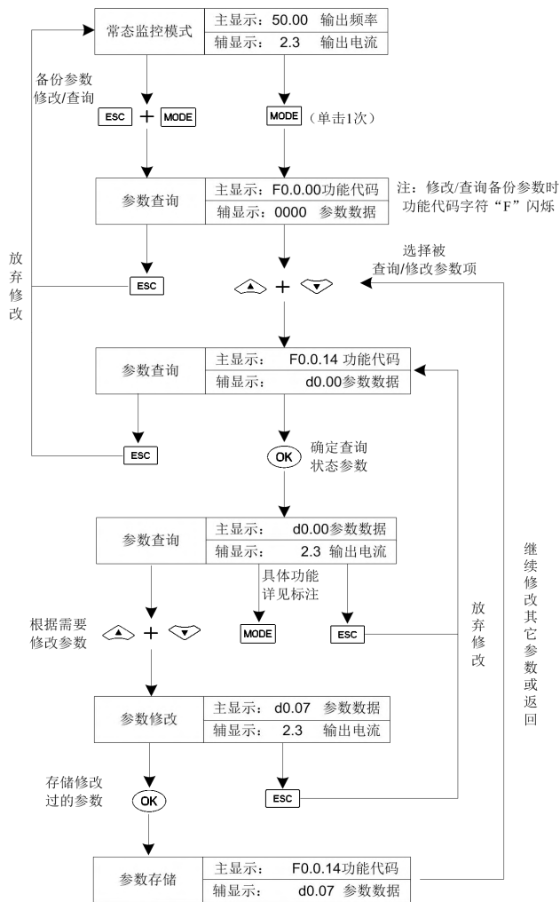
图 5-3 参数查询与修改示意图
