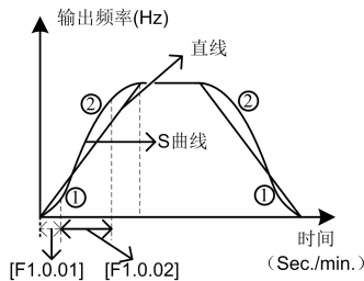
图 7-24 加减速曲线
