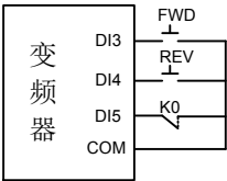
图 7-14-A 三线式运行模式 1
