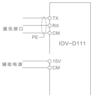
扩展卡配线图
