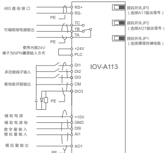
I/O扩展卡配线图
