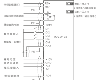
I/O扩展卡配线图
