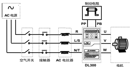
图 3-2 变频器的配线
