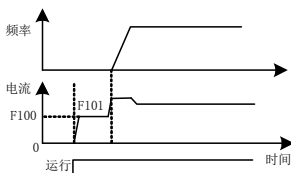
图 6-4 启动预励磁示意图
