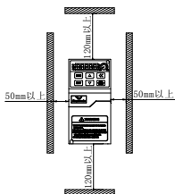
图 2-1-B 安装的间隔距离
