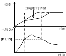
图 6-9 加速电流抑制示意图
