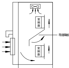
图 2-1-C 多台变频器的安装
