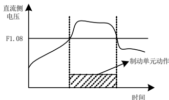
图 6-7 能耗制动
