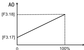
图 6-13 模拟输出
