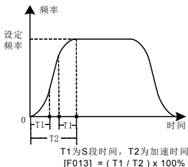
图 6-3 S 曲线加减速示意图
