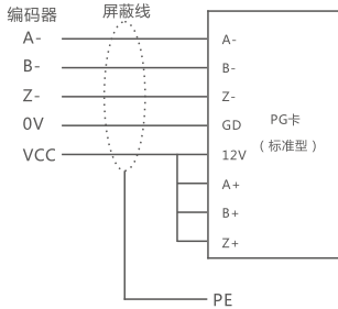
PG卡单端输入配线图
