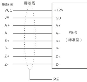
PG卡差分输入配线图
