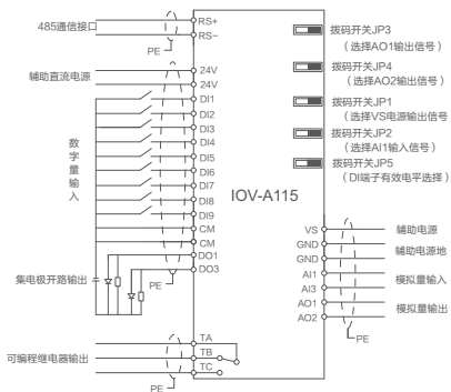
I/O扩展卡配线图
