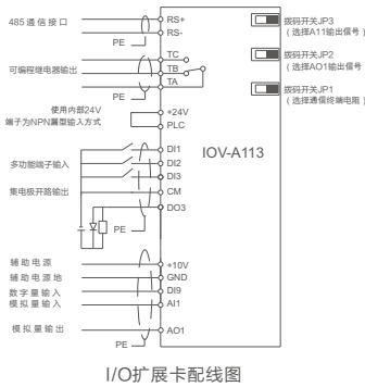
I/O扩展卡配线图
