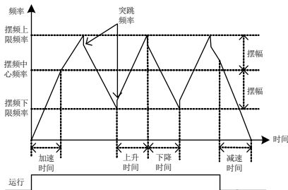
图 6-19 摆频运行示意图
