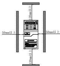
图 2-1-B 安装的间隔距离
