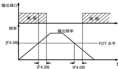
图 6-16 频率水平检测信号 (FDT)
