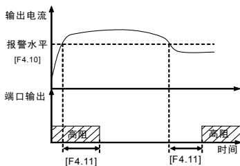
图 6-17 过载报警
