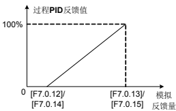
图 7-53 过程 PID 反馈值对应关系示意图
