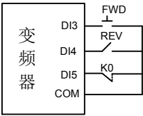
图 7-14-B 三线式运行模式 2
