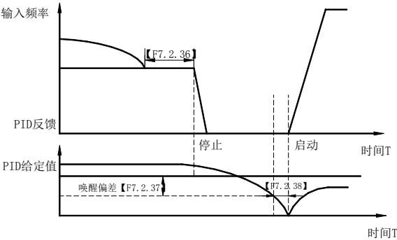
图 7-59 PID 睡眠功能示意图
