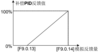
图 7-66 补偿 PID 反馈值定义示意图
