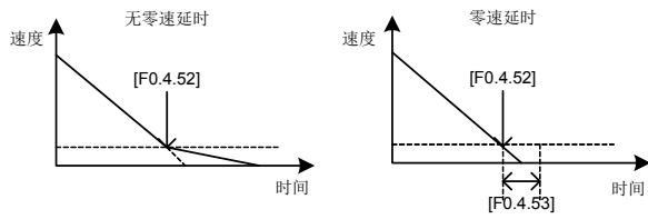
图 7-23 有无零速延时对比图
