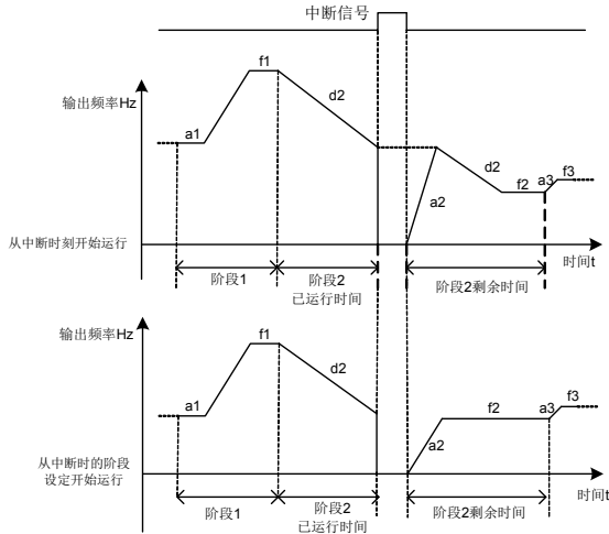
图 7-49 断点恢复示意图
