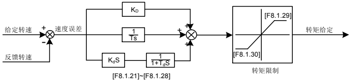
图 7-60 转速闭环框图
