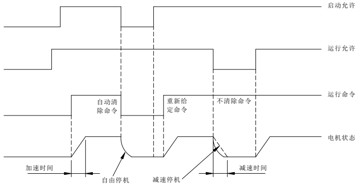
图 7-15 启动过程原理图
