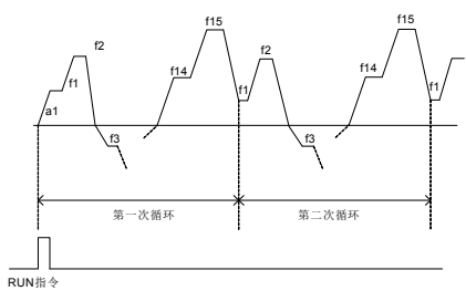
图 7-48-D 简易 PLC 运行连续循环模式
