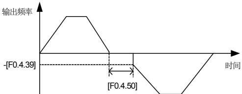
图 7-22 起动频率正反转切换示意图
