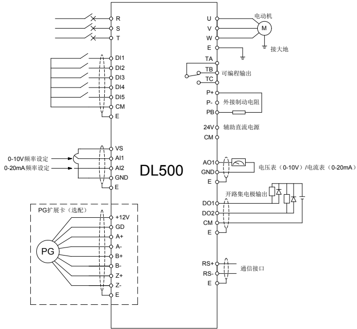
图 4-2 DL500 系列变频器基本接线图
