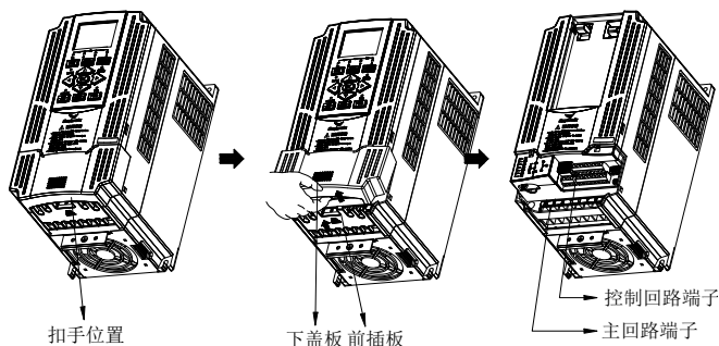
图 3-4 塑壳盖板的拆卸安装示意图
