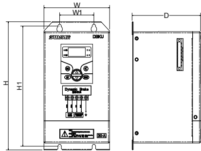
图 12-3 安装尺寸图
