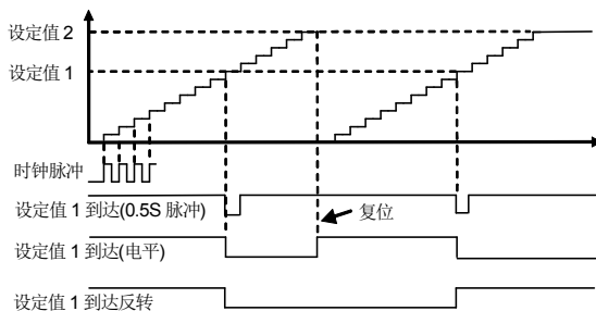
图 7-42-A 计数器功能 1
