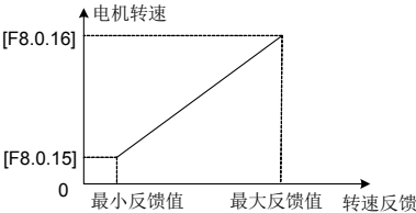
图 7-62 转速反馈值和电机转速对应关系图
