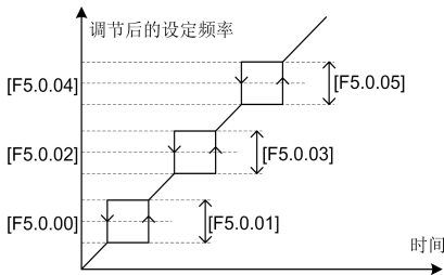
图 7-40 跳跃频率输出示意图
