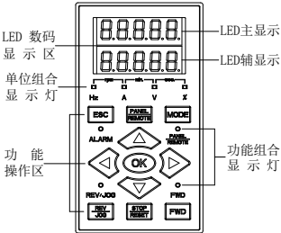
图 5-1-B 双行 LED 标准操作面板
