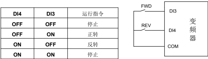
图 7-13-A 两线式运行模式 1
