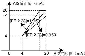
图 7-70-B AI2 增益矫正曲线
