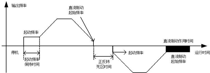
图 7-20 停机直流制动示意图
