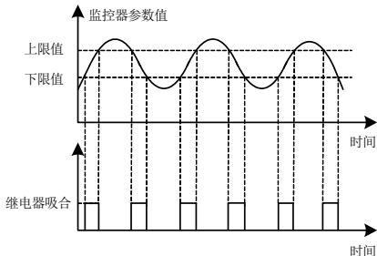
图 7-34-C 监控器功能示意图 3
