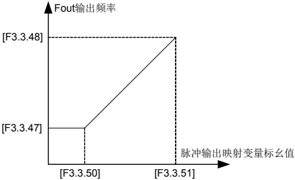
图 7-35 脉冲输出 Fout 特性曲
