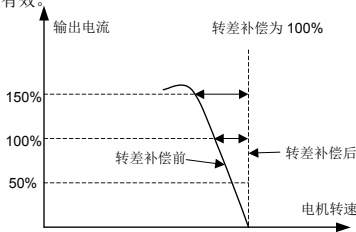
图 7-29 转差频率补偿示意图
