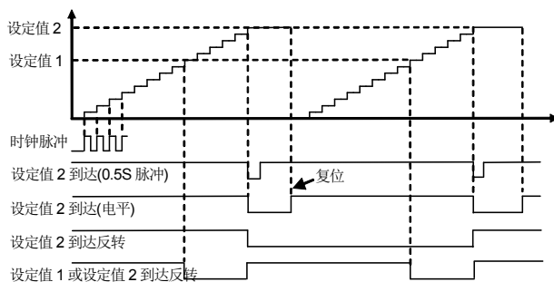
图 7-42-B 计数器功能 2
