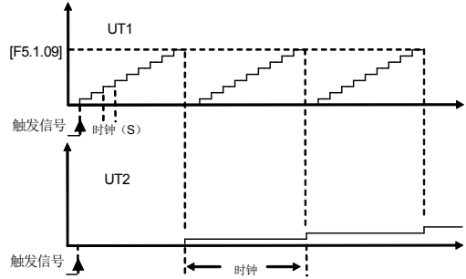
图 7-41-D 定时器 1 (UT1) 的脉冲串接功能 (F5.1.06=10#1; F5.1.07=###3)
