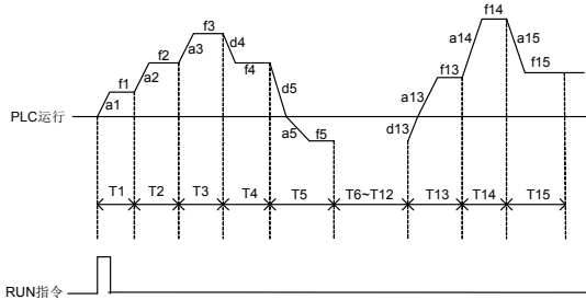
图 7-48-E 简易 PLC 运行保持最终值模式
