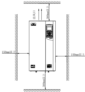
图 3-1-B 安装的间隔距离(37KW 及以上)
