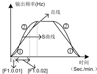
图 7-24 加减速曲线
