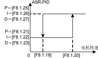
图 7-63-A 双 PID 参数（滞环切换）
