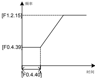
图 7-17 启动频率示意图
