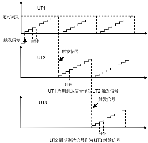
图 7-41-E 定时器 (UT1、UT2、UT3) 的触发串接功能
