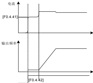
图 7-18 启动预励磁输出
