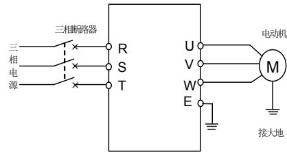
图 5-4 SVC 运行接线
