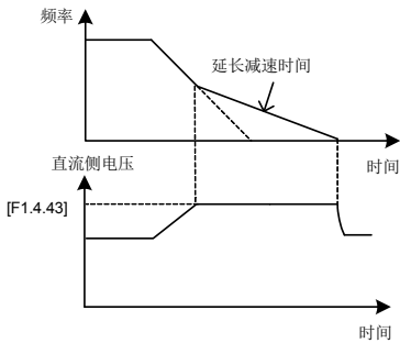
图 7-31-B 减速过程的过压抑制
