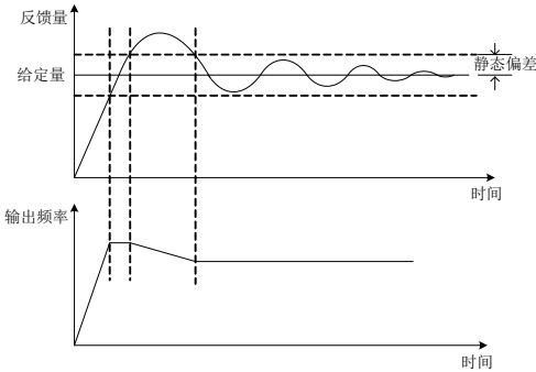
图 7-56 静态偏差示意图
