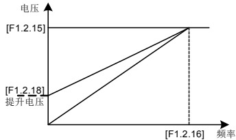
图 7-27-B 恒转矩曲线转矩提升示意图
