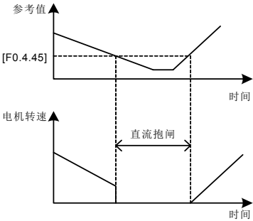
图 7-19 直流抱闸示意图
