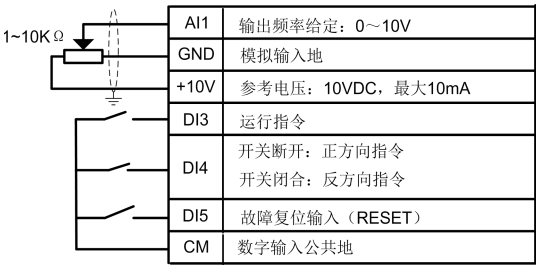
图 7-2-A 两线控制一 AI1 设定接线
