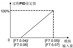
图 7-52 过程 PID 设定值定义示意图
