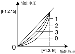
图 7-26 V/F 曲线
