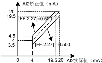
图 7-70-A AI2 零偏矫正曲线
