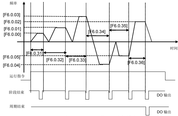
图 7-48-C 简易 PLC 运行单循环停机模式
