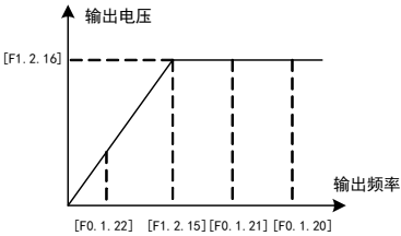
图 7-10 频率参数定义示意图
