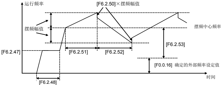
图 7-50 摆频运行示意图
