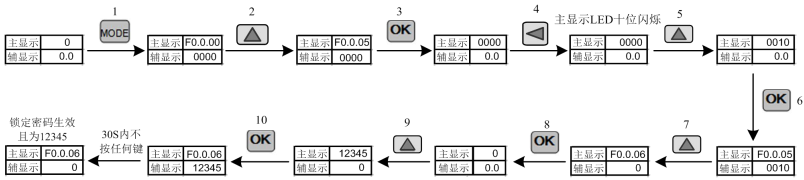
图 7-5 参数锁定操作流程
