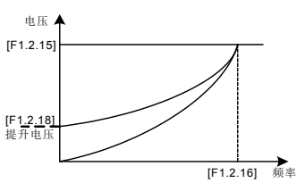
图 7-27-A 降转矩曲线转矩提升示意图
