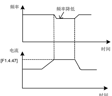
图 7-32-B 限流调节示意图
