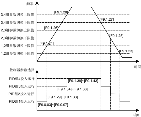
图 7-67 补偿 PID 参数切换示意图
