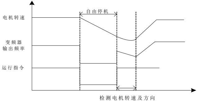
图 7-16 转速跟踪启动示意图
