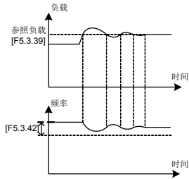
图 7-45 负载动平衡功能示意图
