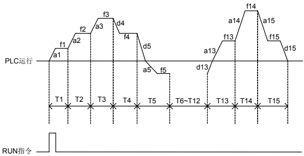
图 7-48-B 简易 PLC 运行单循环模式
