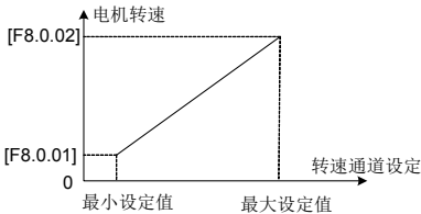
图 7-61 转速设定值和电机转速对应关系图
