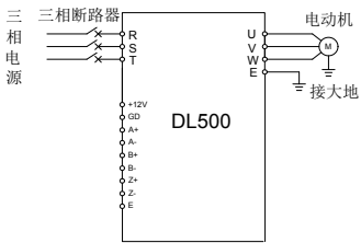
图 5-5 VC 运行接线图
