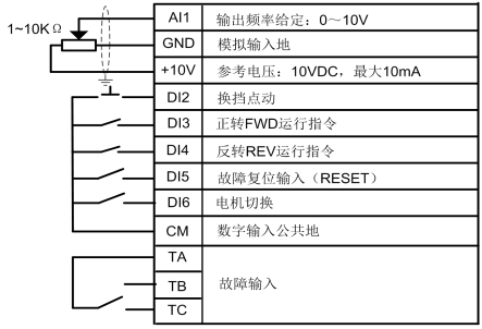
图 7-4 机床主轴驱动宏 AI1 设定接线图
