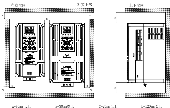
图 3-2 两台变频器（15KW 以上）左右安装尺寸
