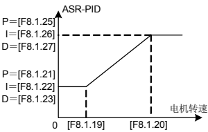
图 7-63-B 双 PID 参数（连续切换）
