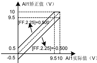
图 7-69-A AI1 零偏矫正曲线
