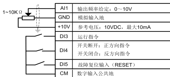
图 7-2-B 两线控制二 AI1 设定接线图
