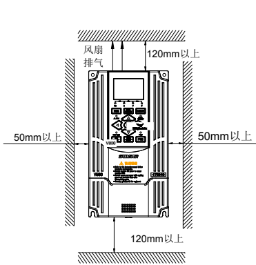
图 3-1-A 安装的间隔距离(30KW 及以下)
