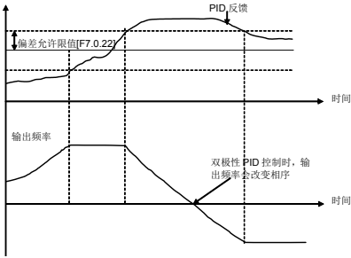
图 7-55-B 双极性 PID 控制方式
