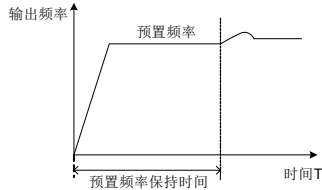
图 7-57 闭环预置频率运行示意图
