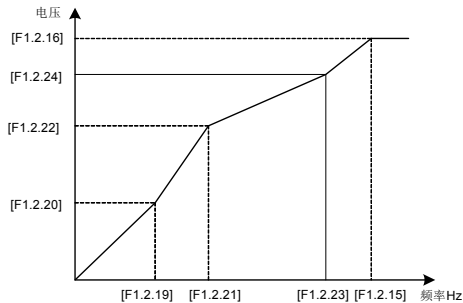
图 7-28 V/F 自定义曲线
