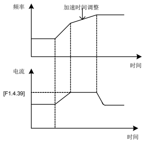
图 7-30 加/减速电流限制示意图
