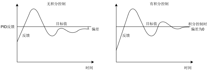
图 7-54 积分控制的作用
