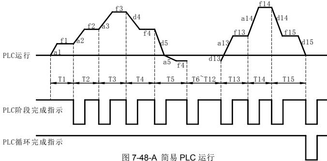
图 7-48-A 简易 PLC 运行
