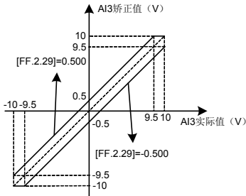
图 7-71-A AI3 零偏矫正曲线
