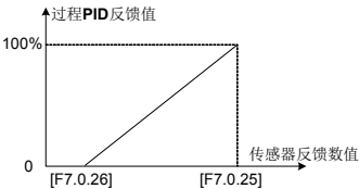
图 7-58 反馈百分比与对应传感器数值的范围曲线
