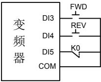
图 7-14-A 三线式运行模式 1
