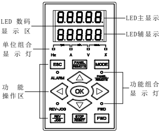
图 5-1-A 双行 LED 小面板
