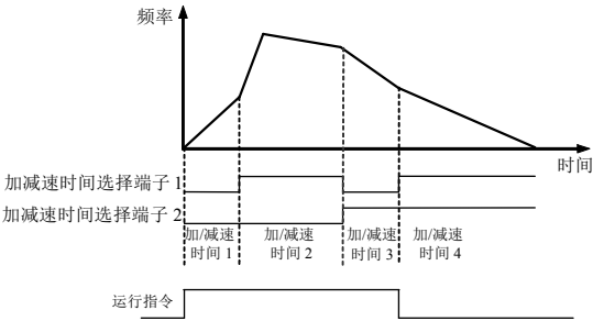
图 7-25 加、减速时间的外部端子选择方式
