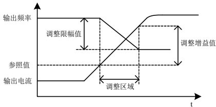
图 7-46 动平衡变量设置示意图
