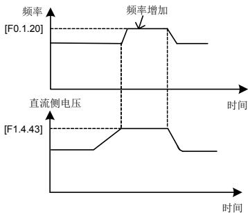
图 7-31-A 稳定运行过程的过压抑制
