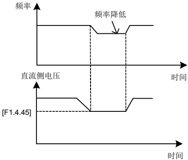
图 7-32-A 欠压调节示意图
