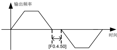
图 7-21 正反转过渡死区示意图
