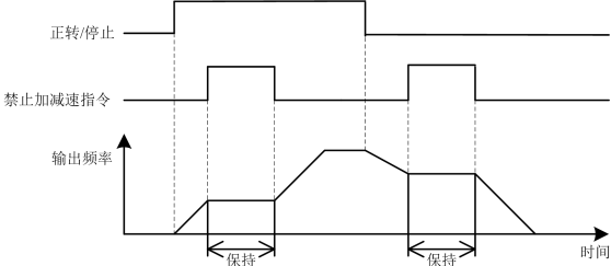
图 7-33 禁止加减速示意图
