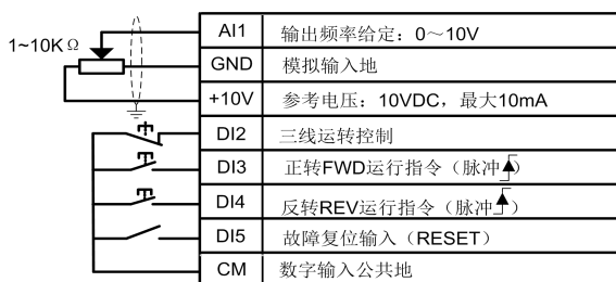
图 7-3 三线控制一/AI1 设定接线图
