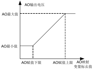
图 7-39AO 输出特性曲线
