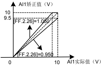
图 7-69-B AI1 增益矫正曲线
