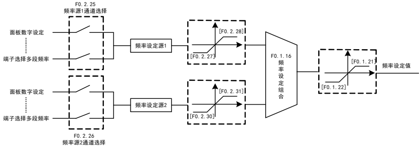
图 7-8 频率设定通道结构示意图
