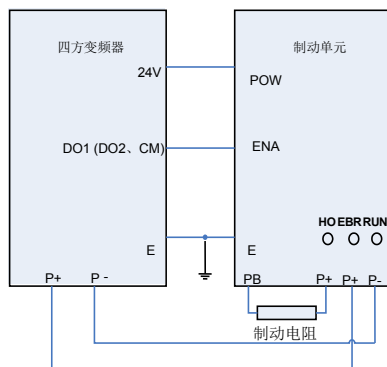
图 12-4 接线示意图
