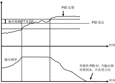
图 7-55-A 单极性 PID 控制方式
