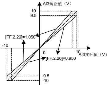
图 7-71-B AI3 增益矫正曲线
