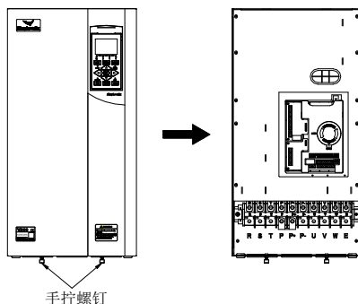
图 3-5 钣金盖板的拆卸安装示意图
