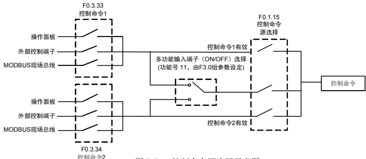
图 7-7 控制命令源选择示意图
