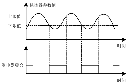
图 7-34-A 监控器功能示意图 1
