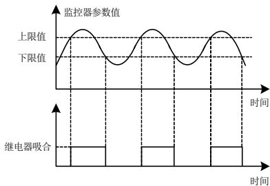
图 7-34-B 监控器功能示意图 2
