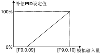
图 7-65 补偿 PID 设定值定义示意图
