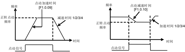
图 7-11 正转点动运行曲线
