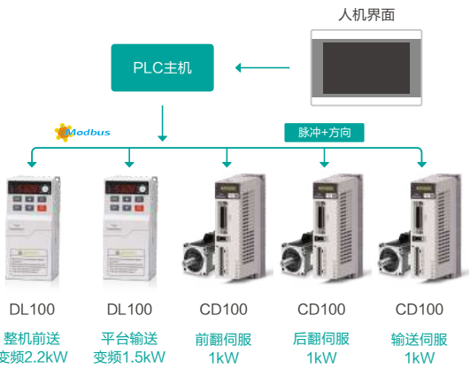
图2 叠被机系统整体结构
