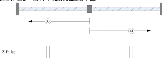
图 5-22 原点回归方式 33/34
