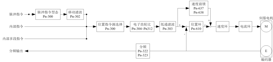
图 5-3 位置控制
