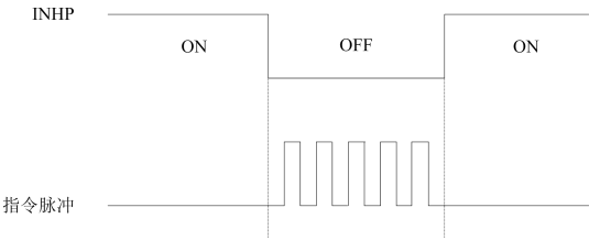
图 5-4 脉冲禁止功能
