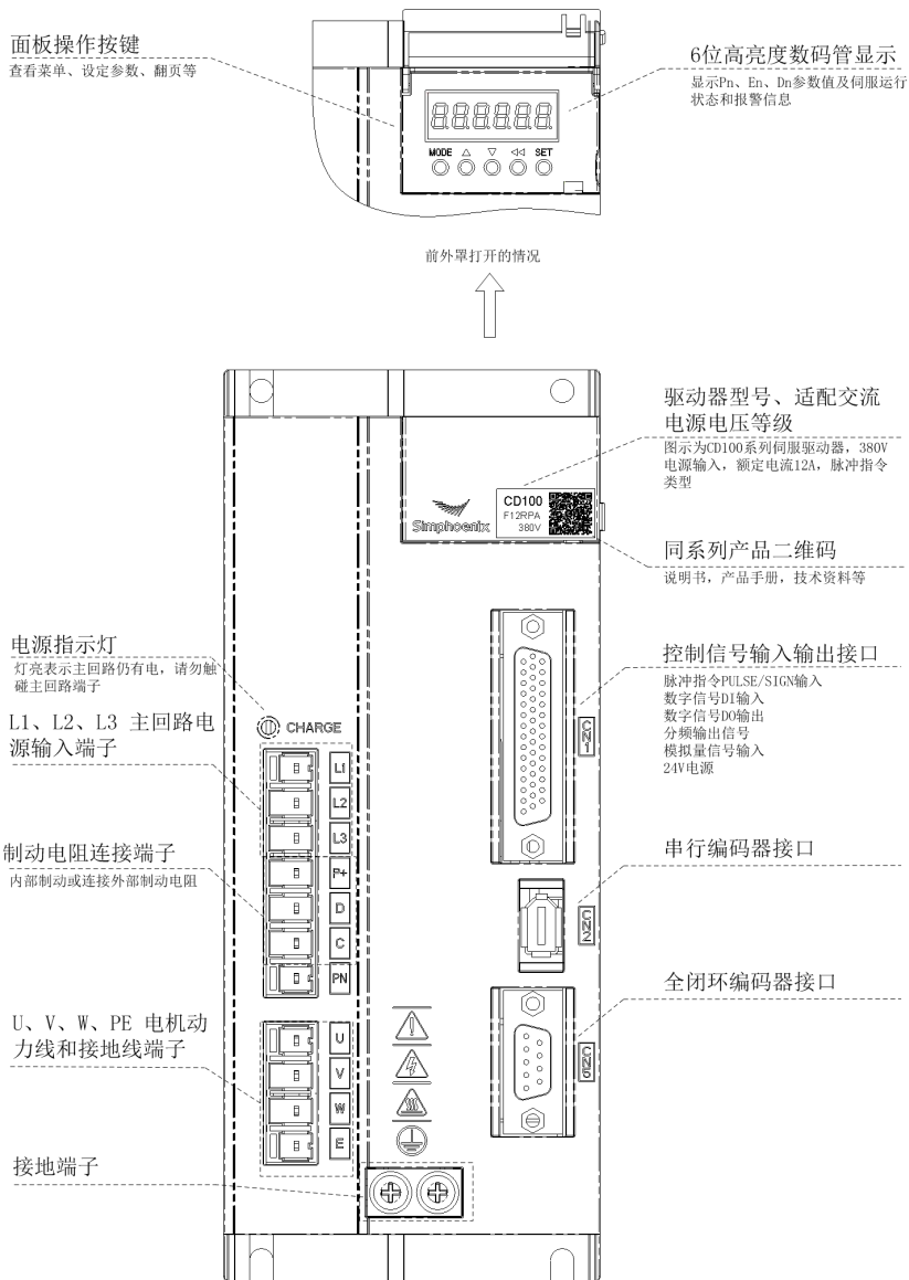
图 1-5 F4R0/F6R5/F8R5/F12R 驱动器各部分名称
