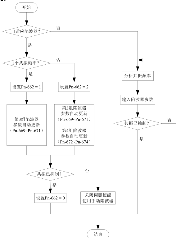
图 6-5 陷波器功能
