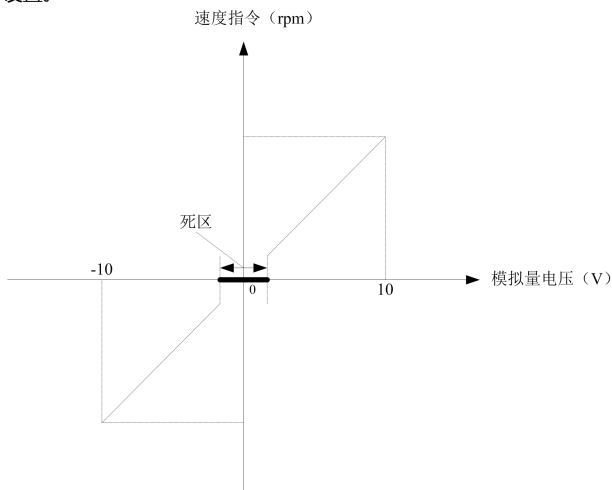
图 5-8 模拟量指令死区
