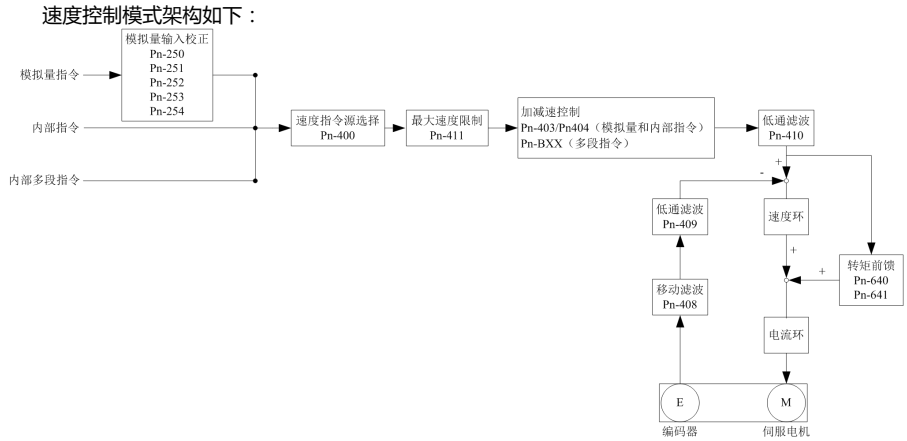
图 5-5 速度控制
