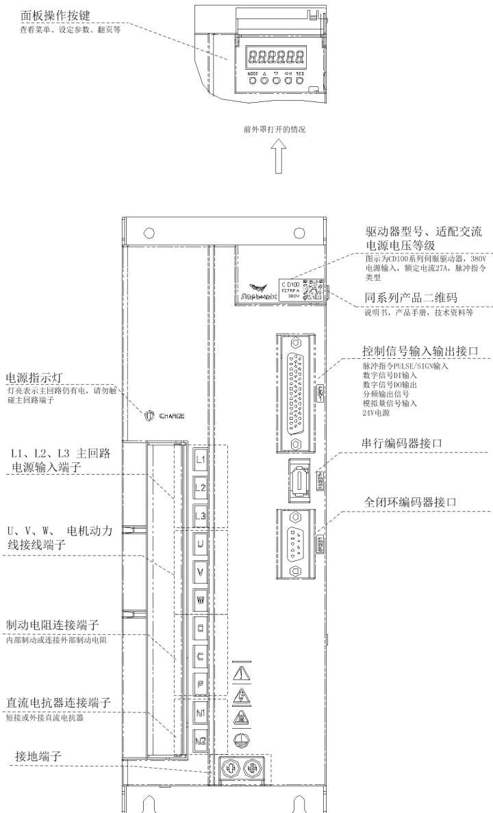
图 1-6 F17R/F22R/F27R 驱动器各部分名称
