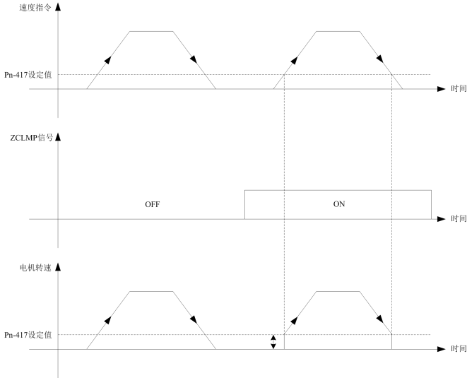
图 5-9 零速箝位
