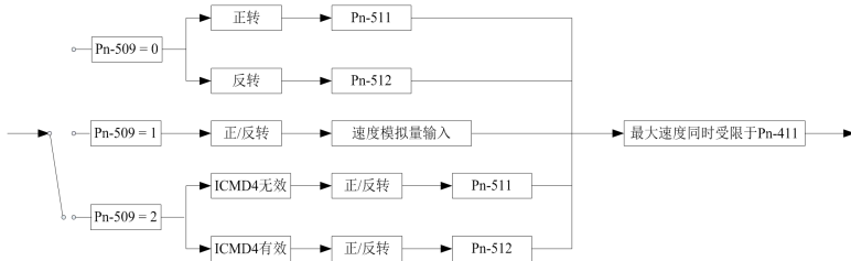
图 5-12 转矩模式下速度限制
