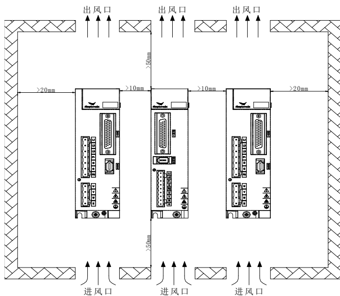
图2-1 伺服驱动器安装方法
