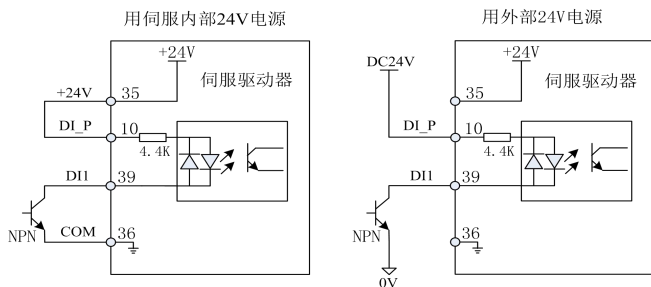
图3-12 上位装置为集电极开路（NPN）输出时的数字输入接线图
