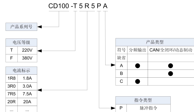
图 1-1 伺服驱动器型号说明
