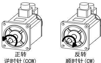
图 5-1 旋转方向定义
