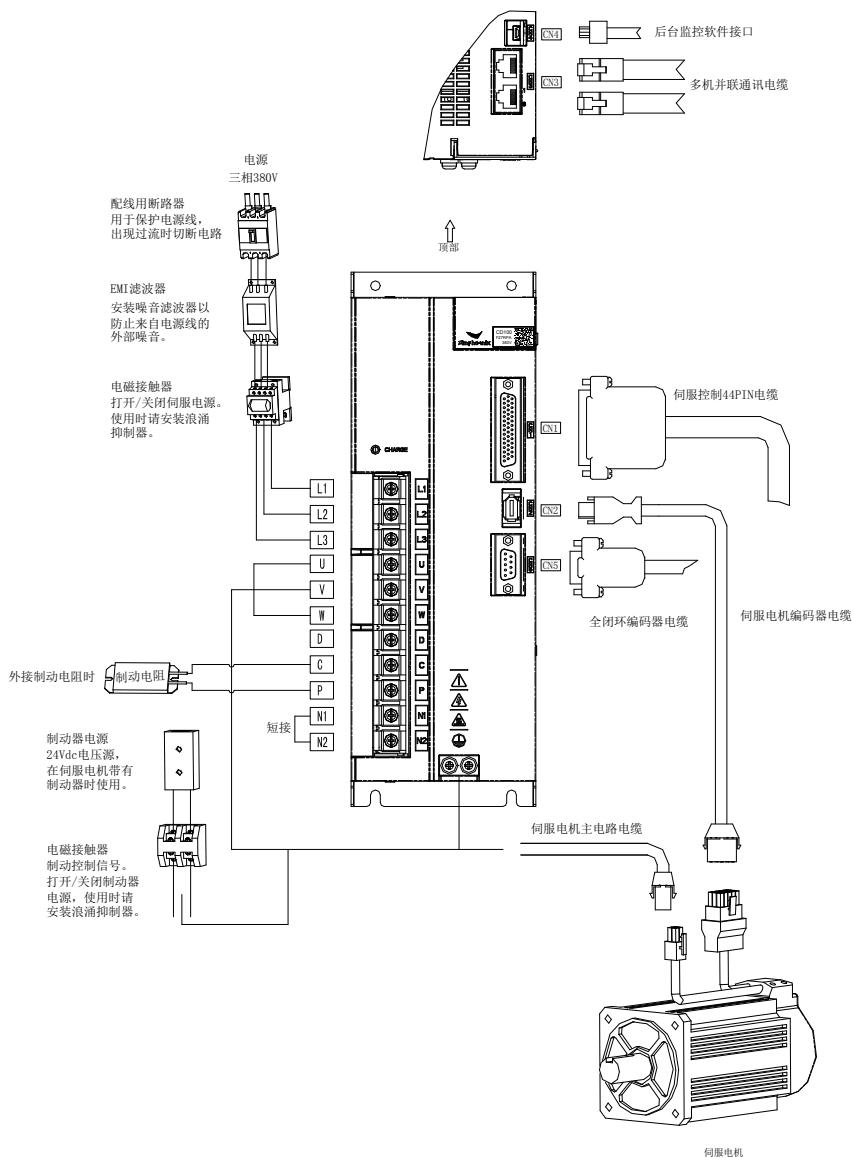
图 3-4 F17R/F22R/F27R 伺服驱动器配线图
