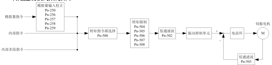
图 5-10 转矩控制
